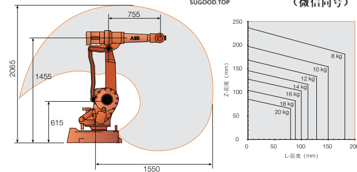
IRB 2400-10, IRB 2400-16
