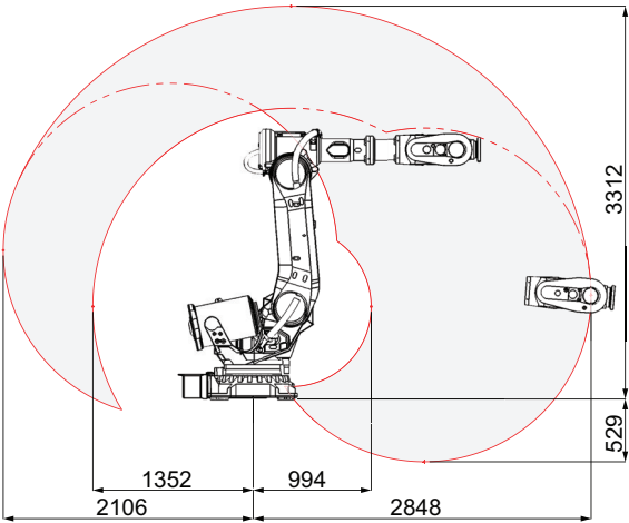
IRB 6700-155/2.85, 工作范围图例
