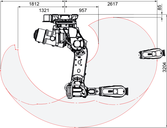
IRB 6700Inv-300/2.60, 工作范围图例
