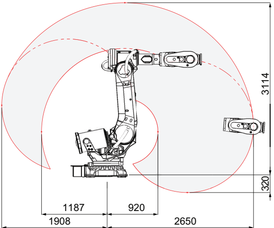
IRB 6700-235/2.65, 工作范围图例
