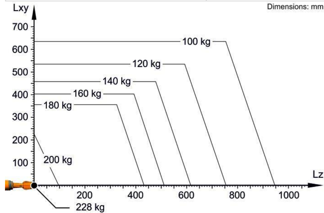
KR 180 R3500-2 K 负载图
