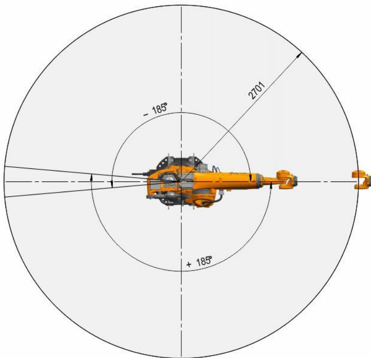
KR 300 R2700-2 F 工作空间, 整体
