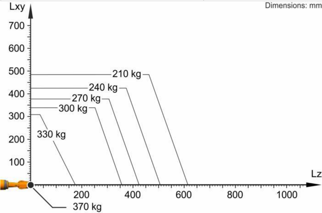
KR 300 R2700-2 F 负载图
