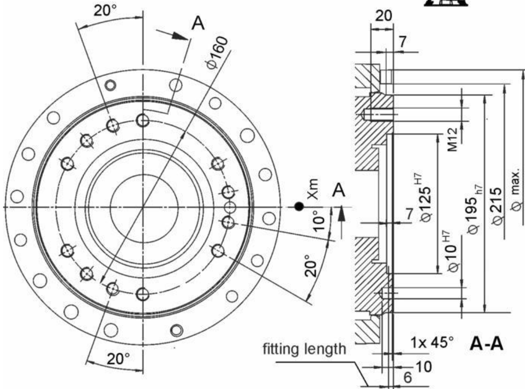
连接法兰
