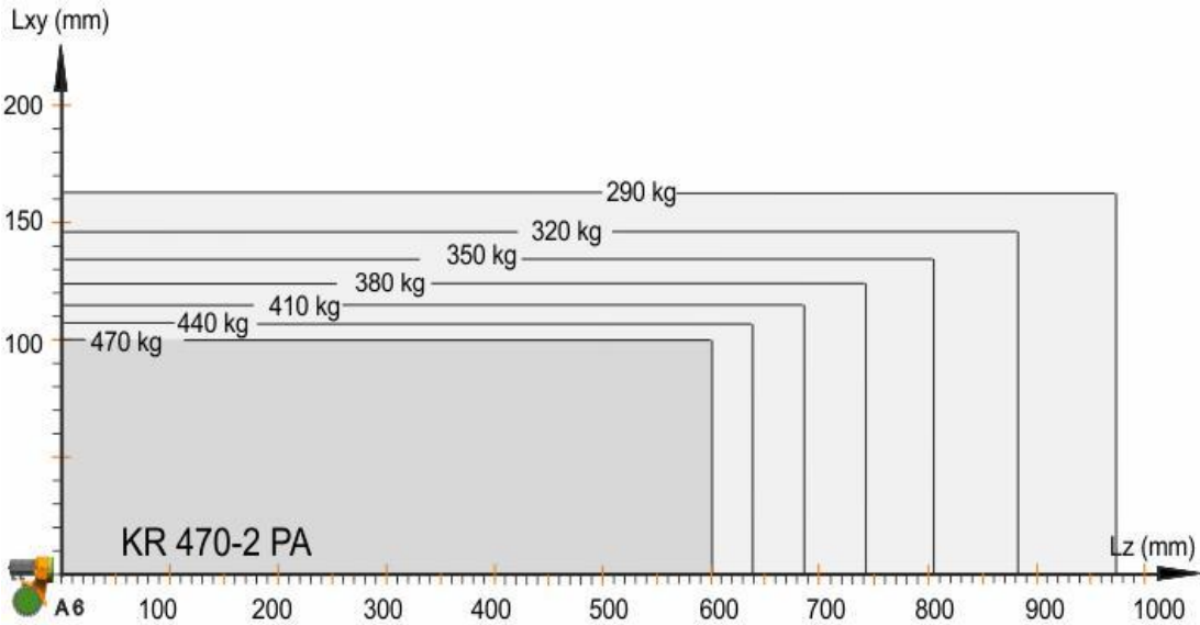
KR 470-2 PA 负载能力图
