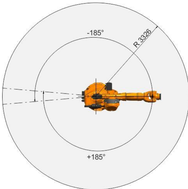
工作区域，总视图，KR 480 R3330 MT
