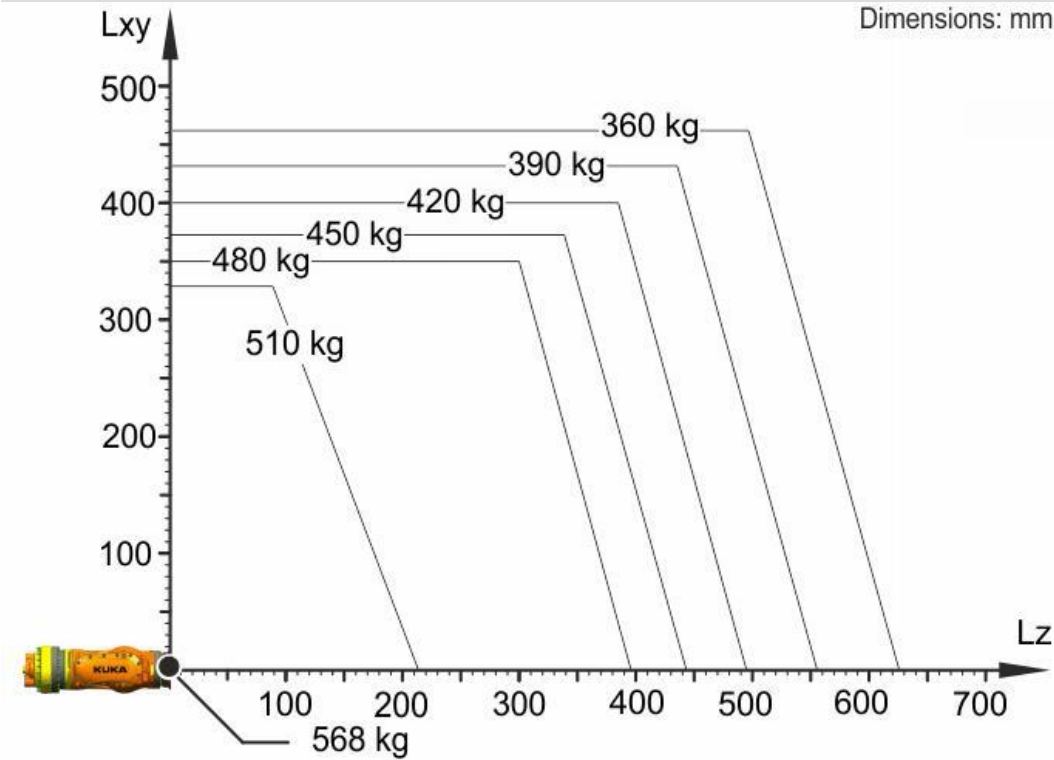
KR 480 R3330 MT 负载能力图
