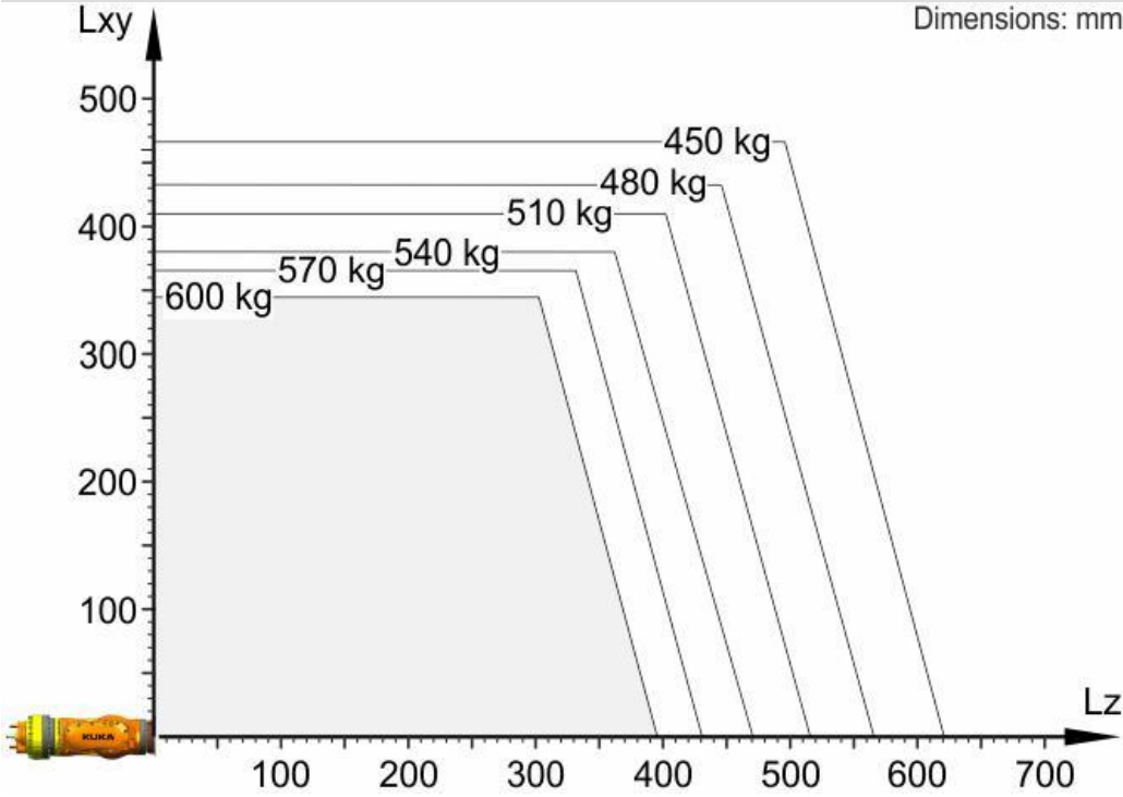
KR 600 R2830 F 负载图
