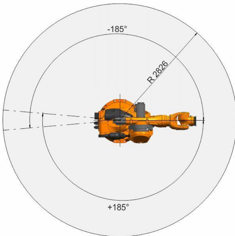
工作空间，总视图，KR 600 R2830 F
