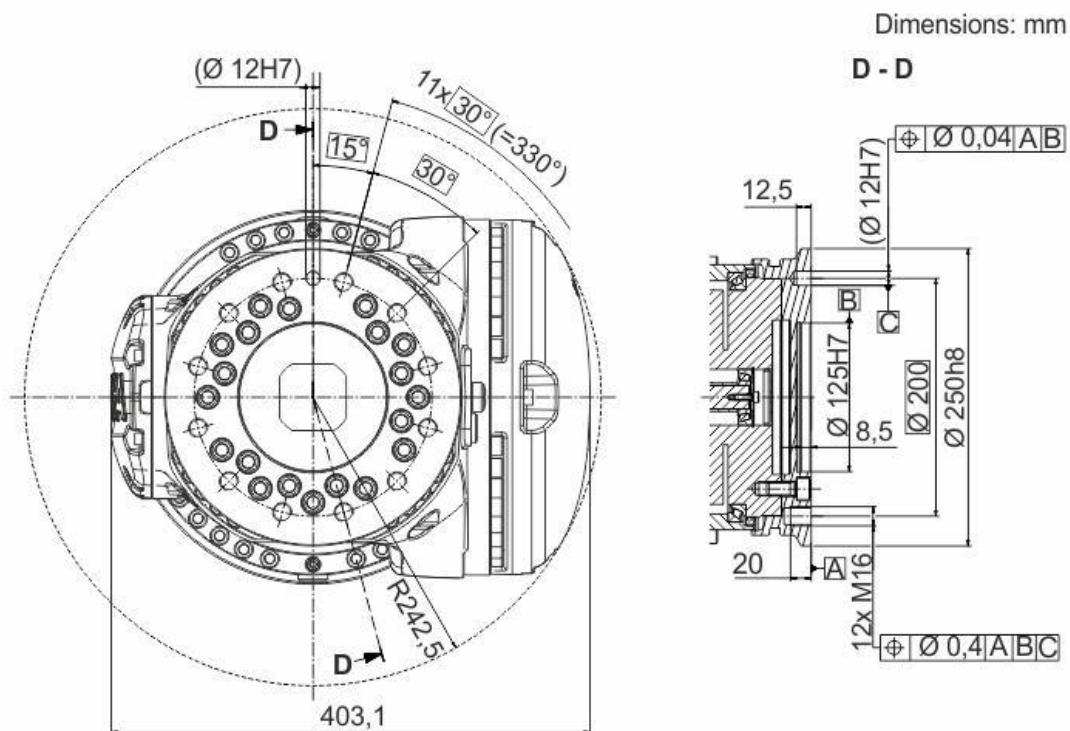
连接法兰 ZH800
