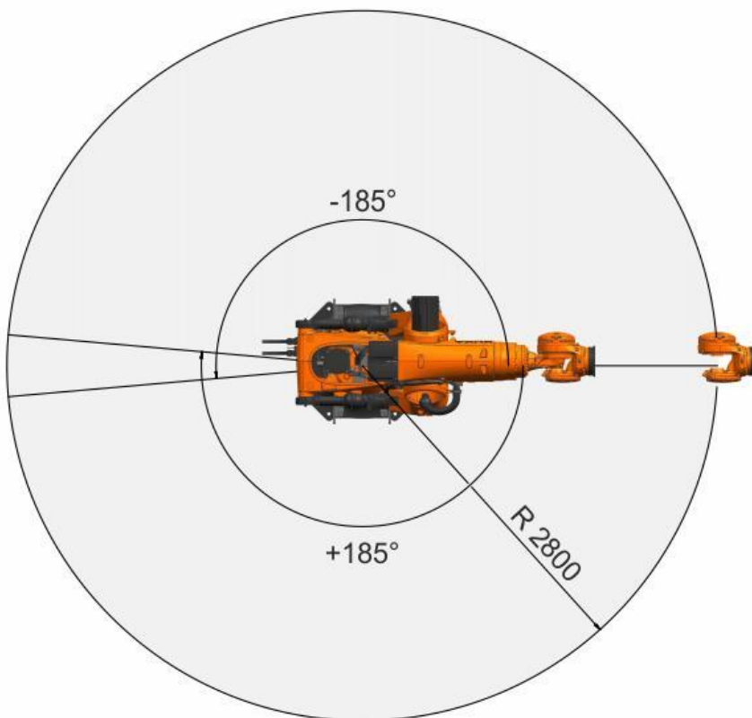
KR 640 R2800-2 工作空间, 总视图
