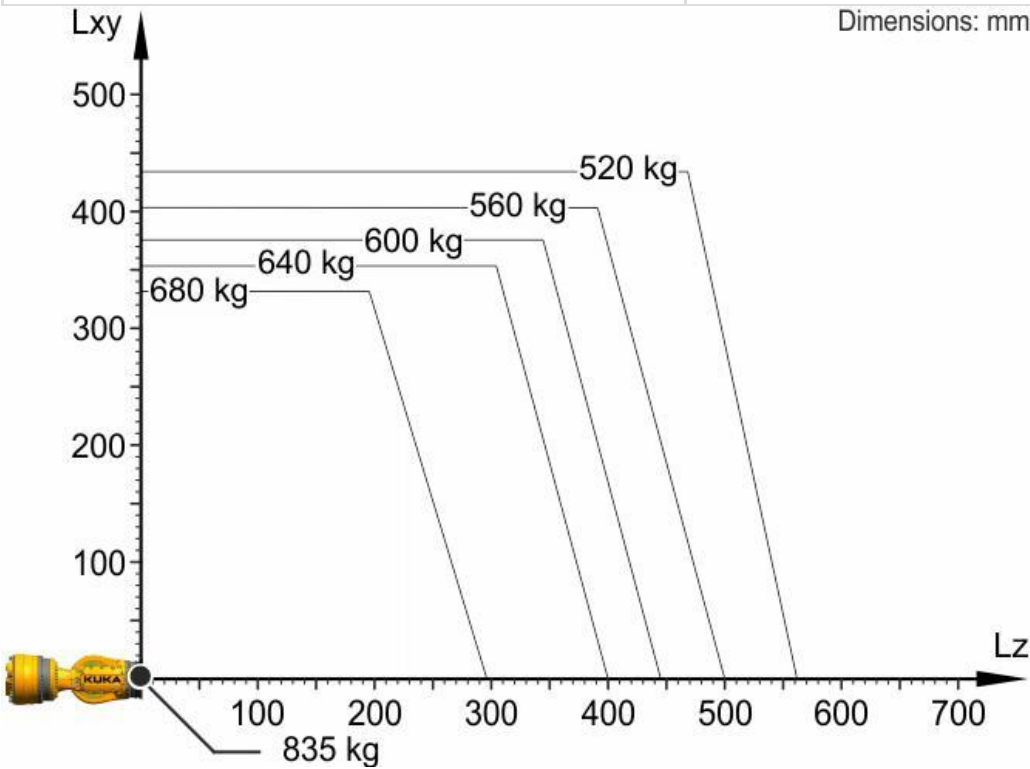
KR 640 R2800-2 负载图
